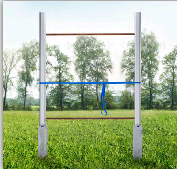
Montage-Tool - Distanzlehren
